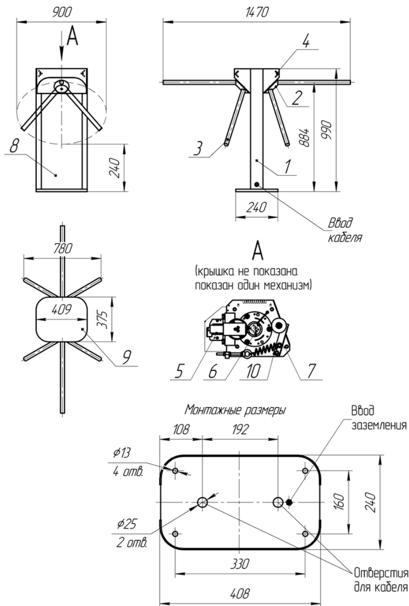
Монтажные (установочные) размеры турникета «Ростов-Дон Т283М1»
